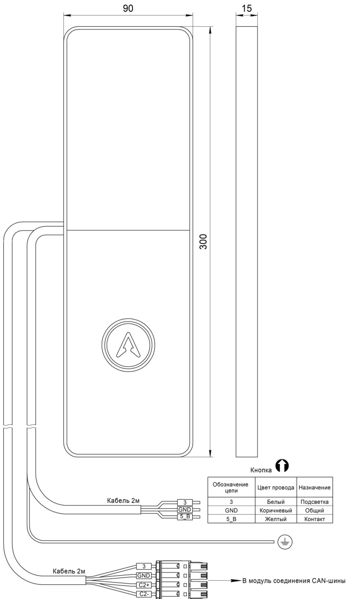
Рис.1 Внешний вид Вызывной пост ОПАЛ НШЕК.468381.056
